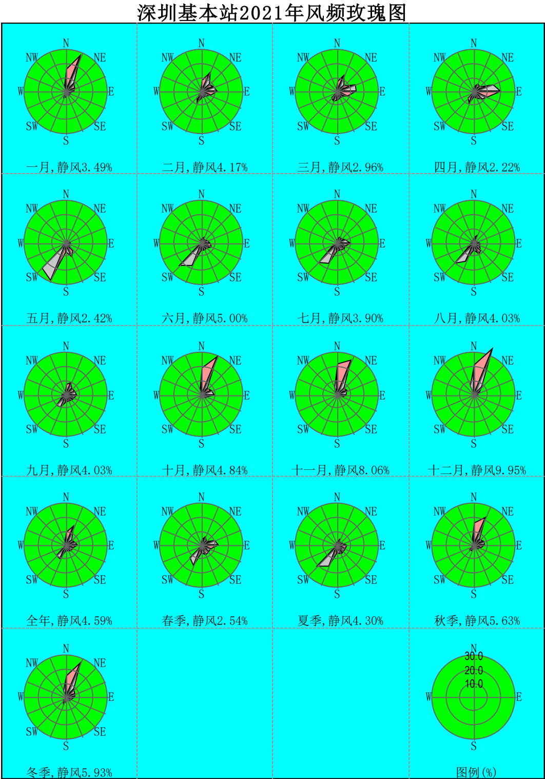
图 5.1-5 风频玫瑰图
