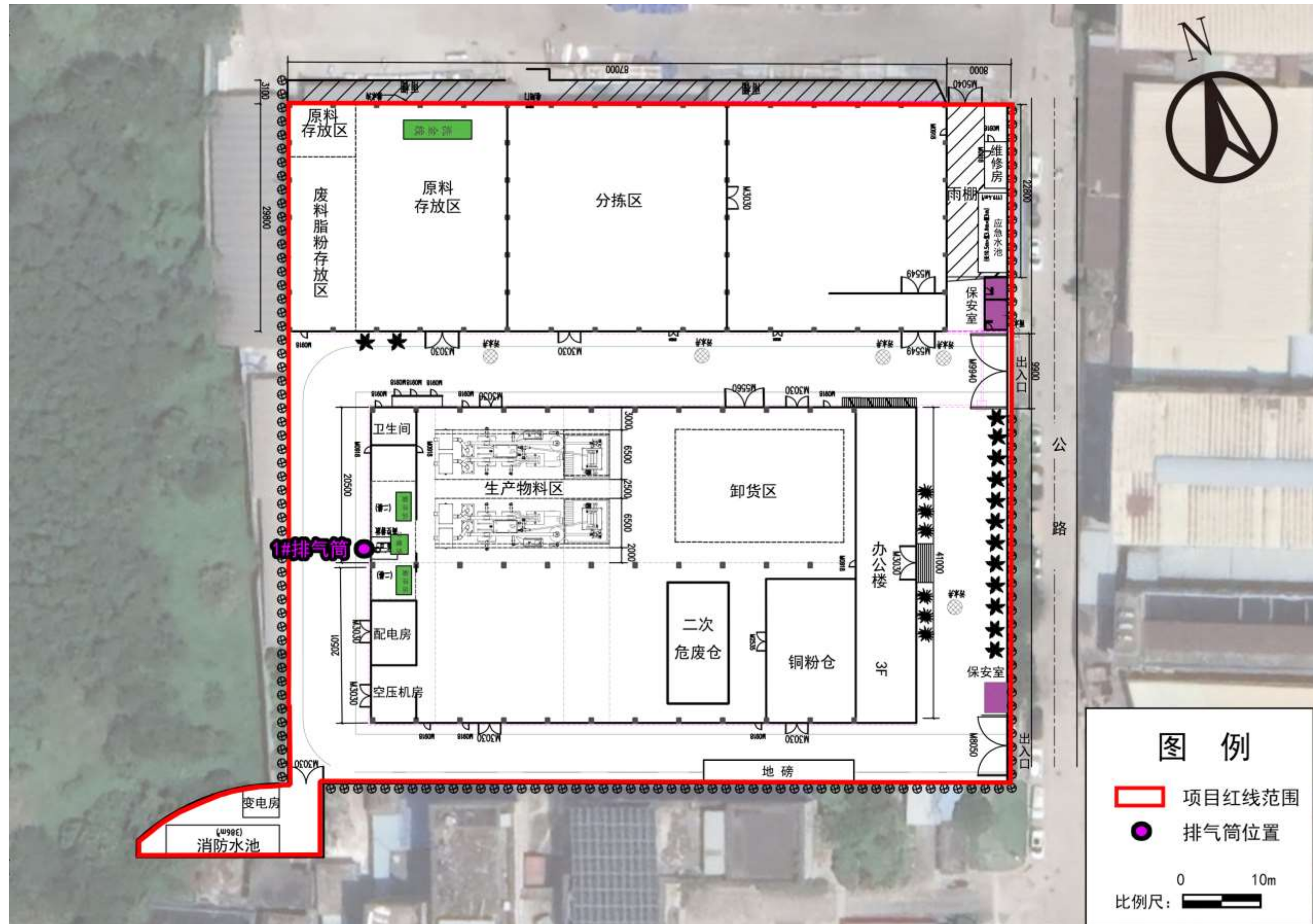
图 3.1-3 本项目实施后厂区平面布置图
