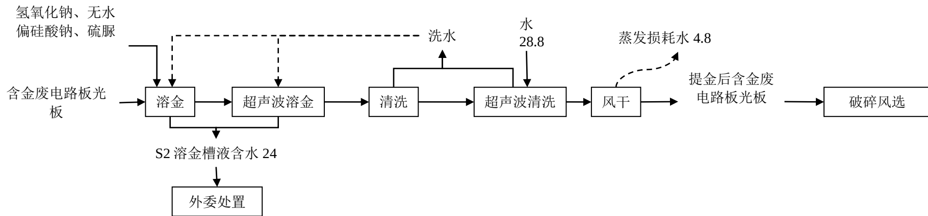
图 3.3-11 废电路板、钻孔粉处理生产线水平平衡示意图 单位: t/a
