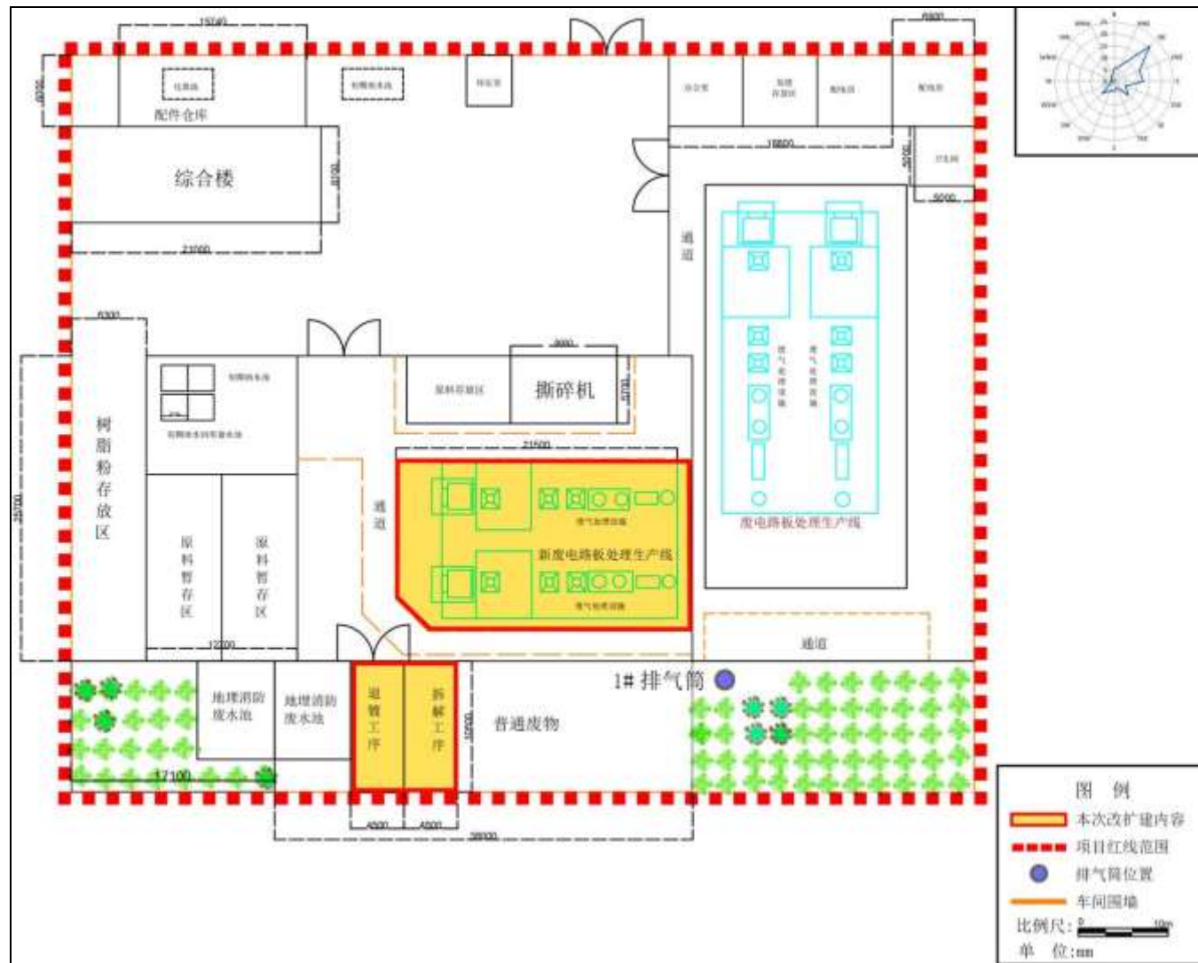
图 2.2-1 现有工程平面图
